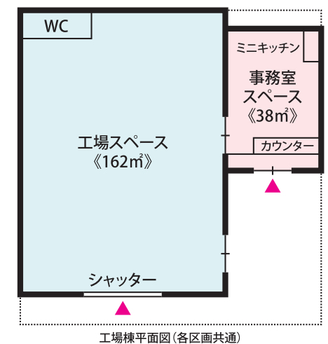
工場棟平面図（各区分共通）
