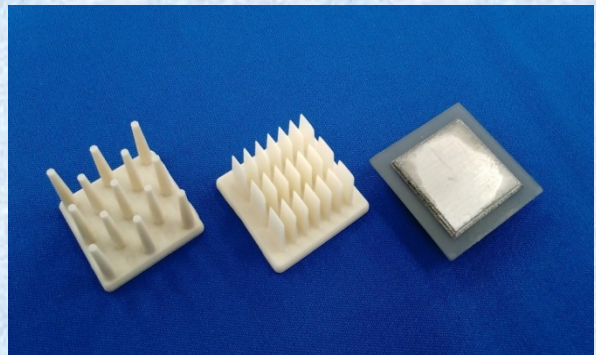
微細形状の CIM 製品サンプル 特徴：耐薬、耐熱、耐磨耗、放熱性向上
